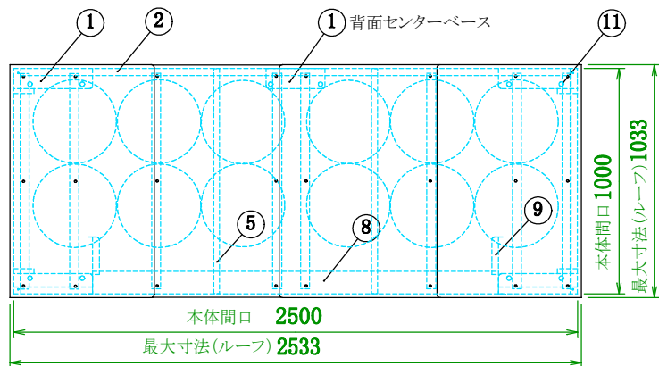
平面図
