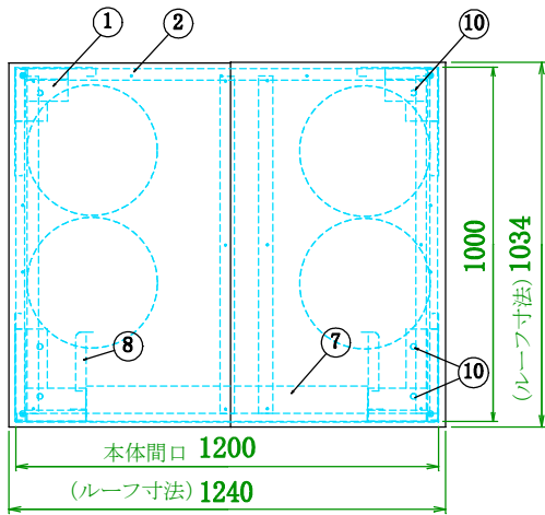
平面図
