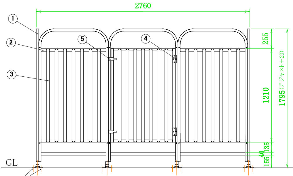
正面図
