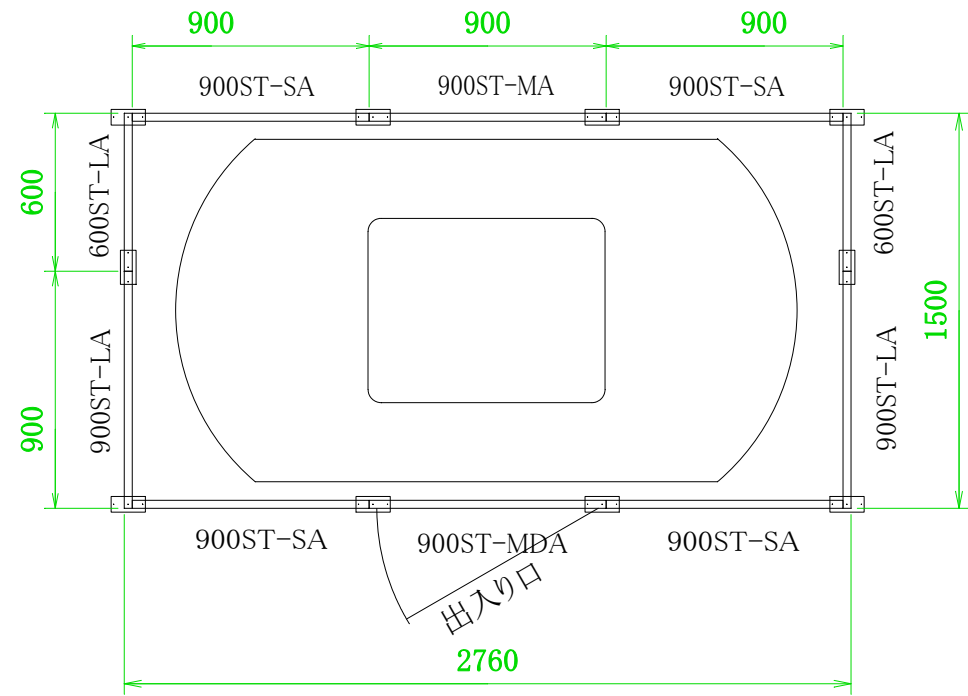
平面図
