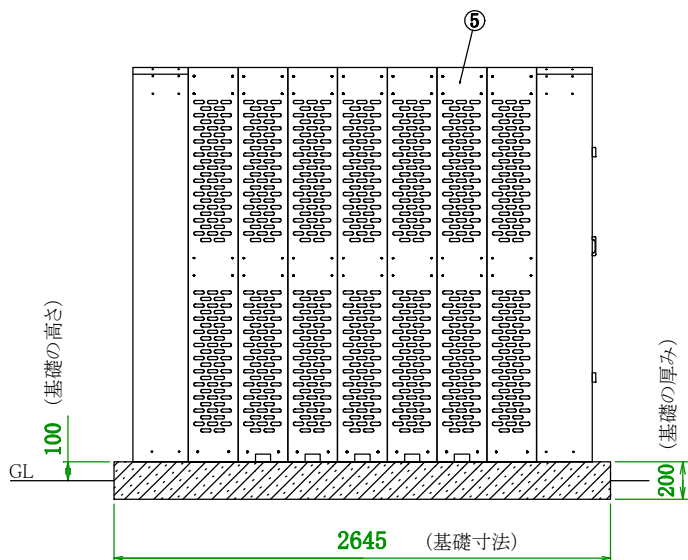
左側面
