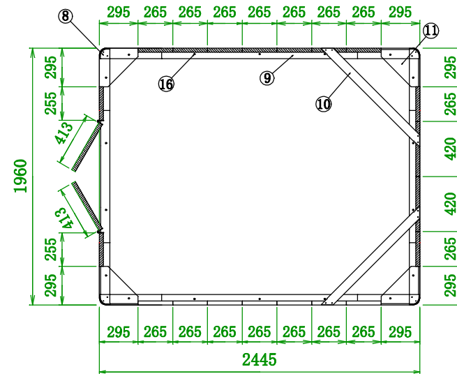
平面
