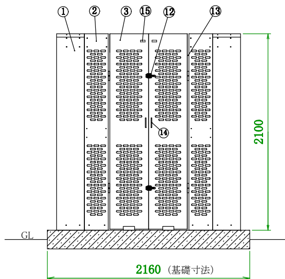
正面
