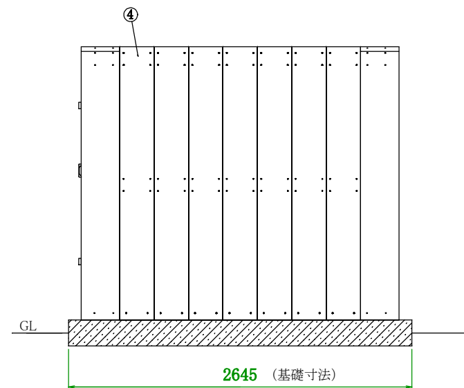
右側面
