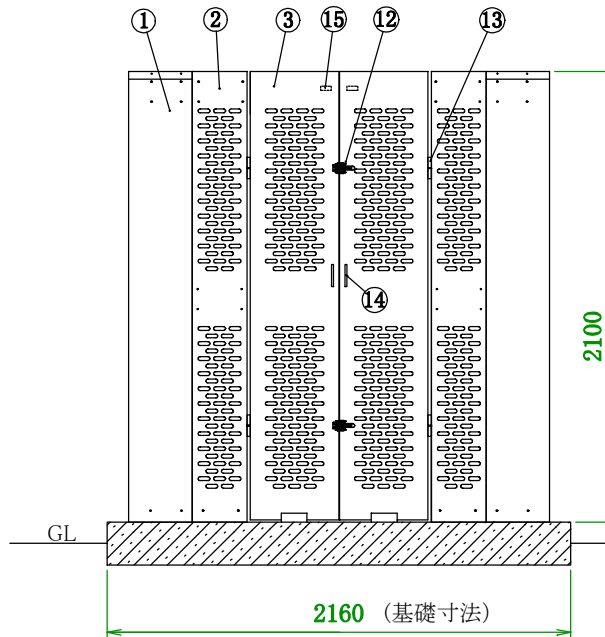
正面
