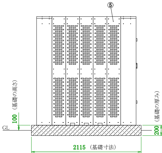
左側面
