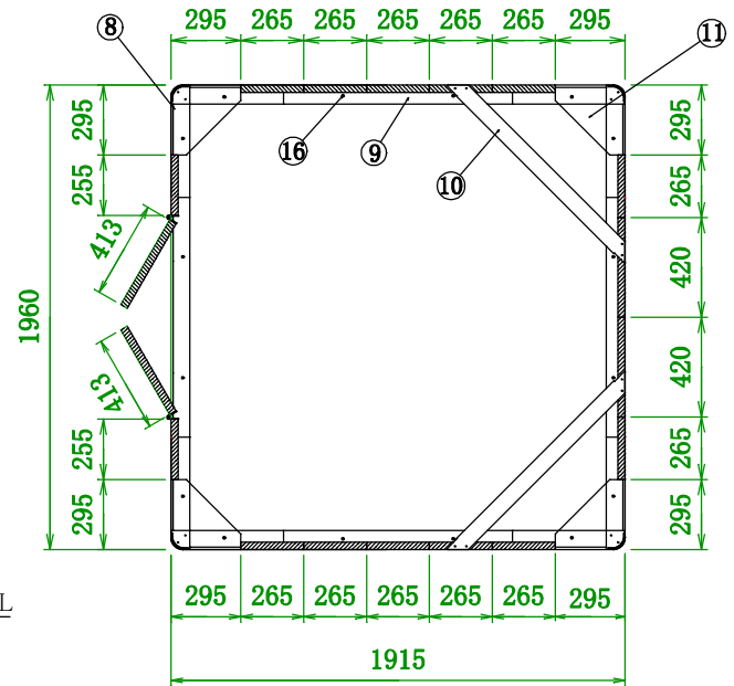
平面
